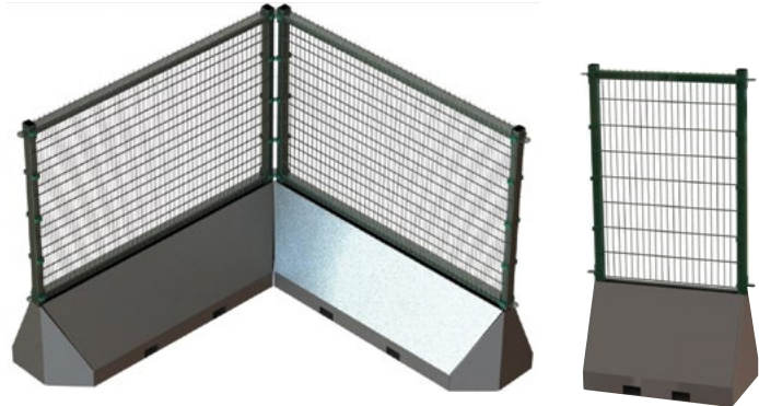
Elementgjerd med Nylofor 2DS og stållplate ved stadion i Salerno, Italia.
